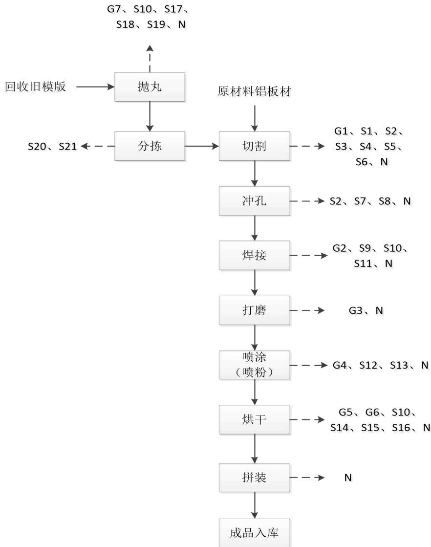
项目生产工艺流程及产污环节图
